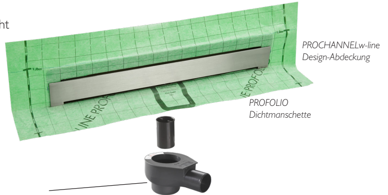
PROCHANNEL Ablauftopf 2, seitlicher Abgang DN 50, Ablaufleistung 0,80 l/s
